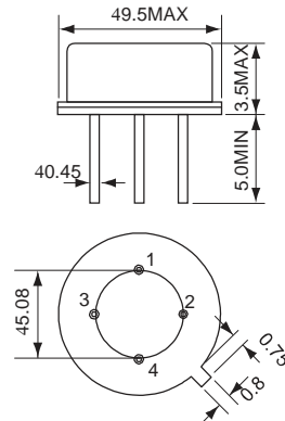
D04 / TO-39
