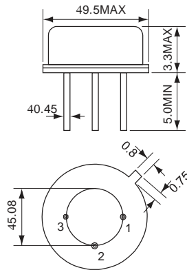
D02 / TO-39
