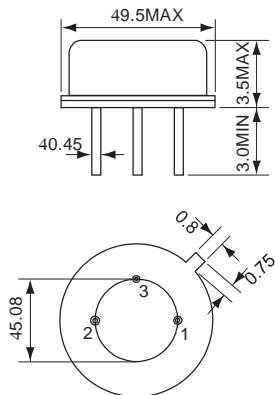
D03 / TO-39
